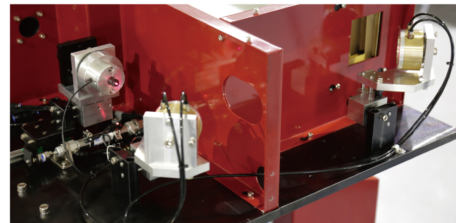
大反射鏡片組，附有自動冷卻系統，散熱性佳，功率衰退少
