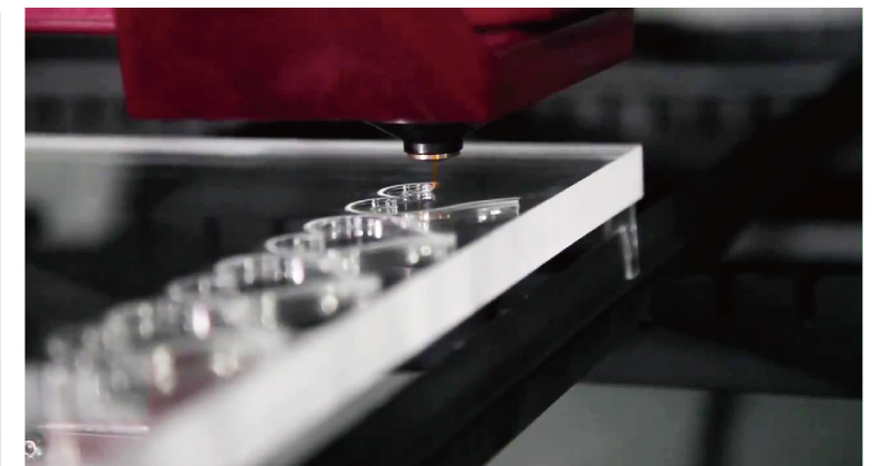
活動輔助夾具 可手動前後調夾具間距 檯面具備六個分區吸著，自動感應分區排煙。 檯面可手動或自動升降，方便大型板材上下料。
