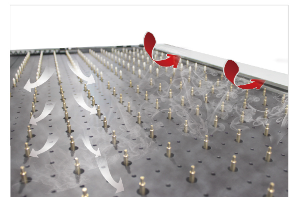
活動輔助夾具 可手動前後調夾具間距 檯面具備六個分區吸著，自動感應分區排煙。 檯面可手動或自動升降，方便大型板材上下料。
