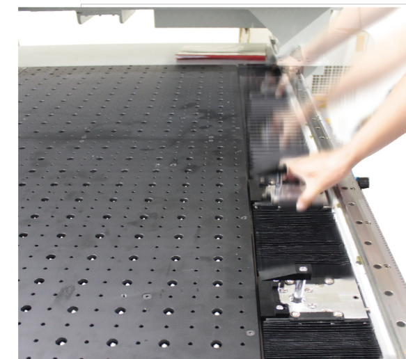
活動輔助夾具 可手動前後調夾具間距 檯面具備六個分區吸著，自動感應分區排煙。 檯面可手動或自動升降，方便大型板材上下料。
