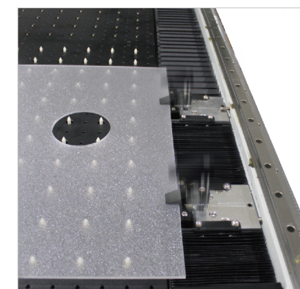
自動夾具系統可針對切割板材厚度變換高度夾持
